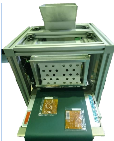
バキュームフィーダー
